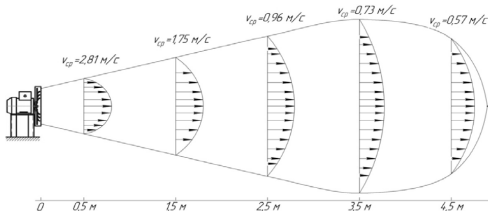
Рис. 3. Средняя скорость напора воздуха осевого вентилятора с центробежными лопатками
