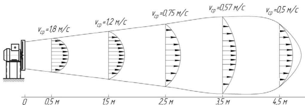
Рис. 2. Средняя скорость напора воздуха осевого вентилятора
