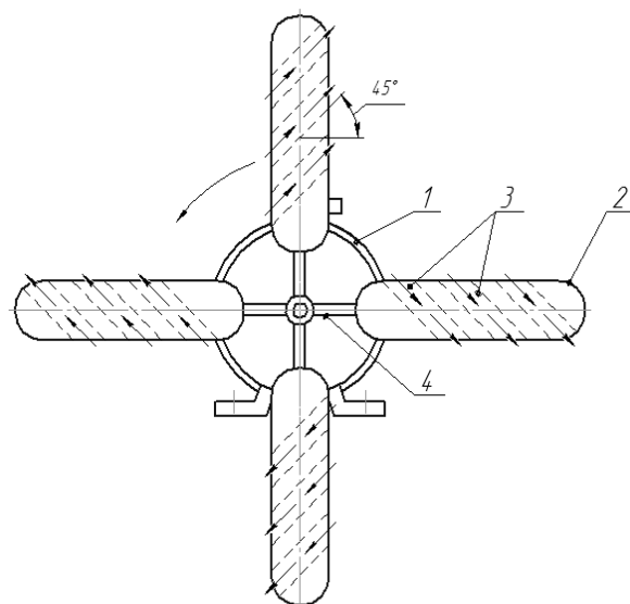
Рис. 1. Осевой вентилятор с центробежными лопатками
