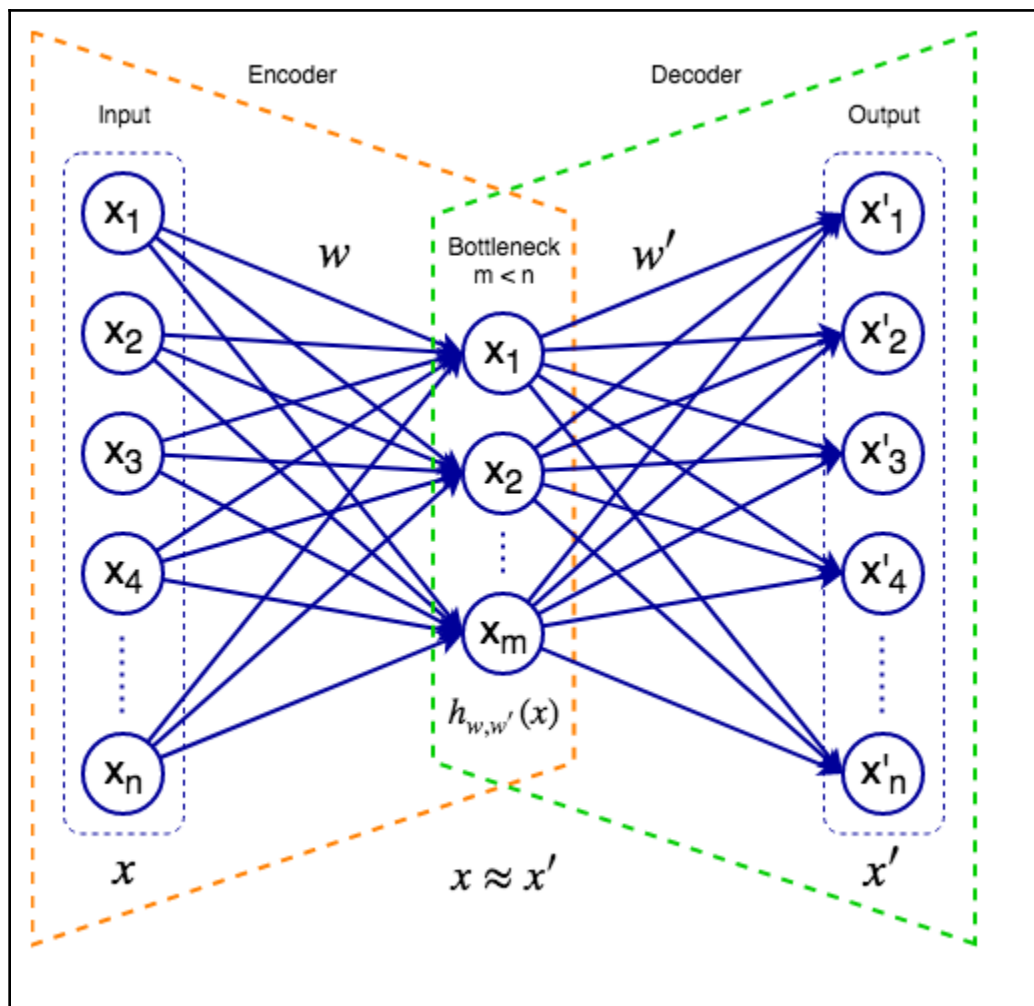
An autoencoder
