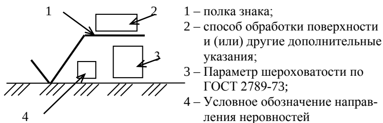
Рисунок 5.4 – Условный знак обозначения шероховатости поверхности
