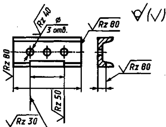
Рисунок 5.7 – Пример обозначения шероховатости на чертеже
