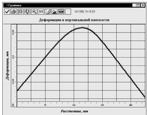
Рисунок 4.8 – Эпюра
